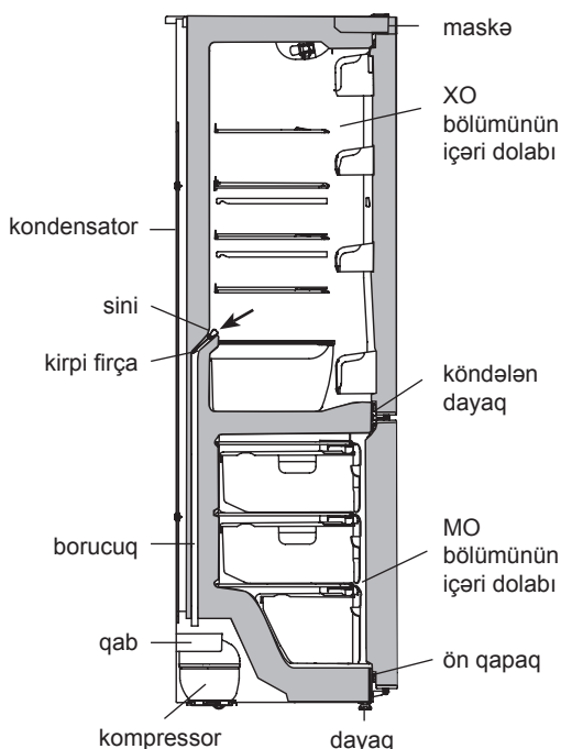
Rəsim 5 — XO bölümünün ərmiş axıntı sularının töküləməsi sxemi
